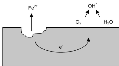
Figure 1 : Processus de corrosion
